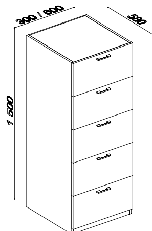
22066 KARTOTÉKA A5 NIZKÁ 300 / 580 / 1500 MM 22067 KARTOTÉKA A5 NIZKÁ 600 / 580 / 1500 MM
