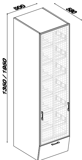
22090 LÉKÁRNA S VÝSUVNÝMI SKLENĚNÝMI DVÍŘKY S AL. RÁMEČKEM 500 / 580 / 1350 MM
