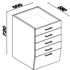
22002 SKŘÍŇKA SPODNÍ SE ZÁSUVKAMI
