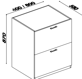
22063 KARTOTÉKA A4 NIZKÁ 400 / 580 / 870 MM 22064 KARTOTÉKA A4 NIZKÁ 800 / 580 / 870 MM
