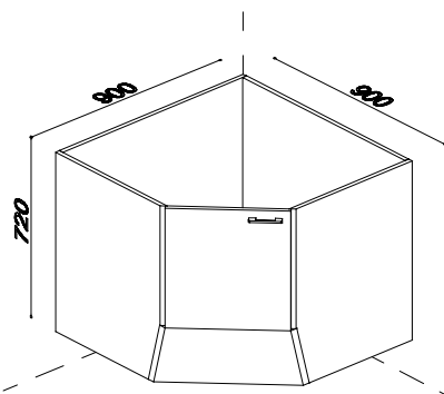
22016 SKŘÍŇKA SPODNÍ ROHOVÁ S DVÍŘKY
