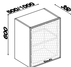
22030 SKŘÍŇKA HORNÍ S VÝKLOPNÝMI SKLENĚNÝMI DVÍŘKY S AL. RÁMEČKEM 500 / 350 / 600 MM 22031 SKŘÍŇKA HORNÍ S VÝKLOPNÝMI SKLENĚNÝMI DVÍŘKY S AL. RÁMEČKEM 1000 / 350 / 600 MM
