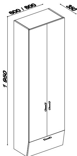
22102 SKŘÍŇ ŠATNÍ S PLNÝMI DVÍŘKY 600 / 350 / 1950 MM
