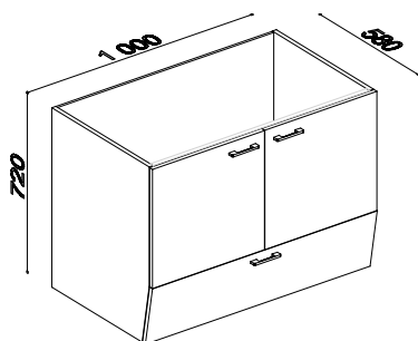
22012 SKŘÍŇKA SPODNÍ POD DVOJDŘEZ S DVÍŘKY
