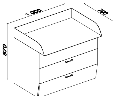
22140 PŘEBALOVACÍ STŮL
