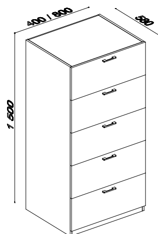
22069 KARTOTÉKA A4 NIZKÁ 400 / 580 / 1500 MM 22070 KARTOTÉKA A4 NIZKÁ 800 / 580 / 1500 MM
