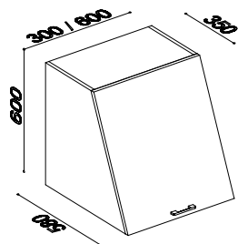
22072 NADSTAVEC NAD KARTOTÉKU A5 300 / 350-580 / 600 MM 22073 NADSTAVEC NAD KARTOTÉKU A5 600 / 350-580 / 600 MM
