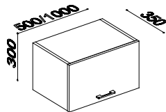
22022 SKŘÍŇKA HORNÍ S VÝKLOPNÝMI PLNÝMI DVÍŘKY 500 / 350 / 300 MM 22023 SKŘÍŇKA HORNÍ S VÝKLOPNÝMI PLNÝMI DVÍŘKY 1000 / 350 / 300 MM
