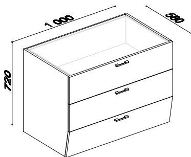
22006 SKŘÍŇKA SPODNÍ SE ZÁSUVKAMI
