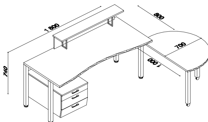
22111 SAMOSTATNÉ PRACOVISTÉ
