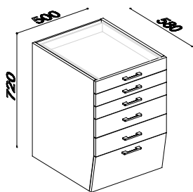
22001 SKŘÍŇKA SPODNÍ SE ZÁSUVKAMI
