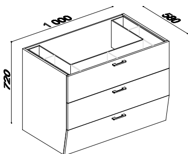
22013 SKŘÍŇKA SPODNÍ POD DŘEZ PŘÍP. DVOJDŘEZ SE ZÁSUVKAMI
