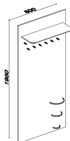
22150 VĚŠÁKOVÁ STĚNA
