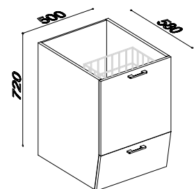
22015 SKŘÍŇKA SPODNÍ PRO KOŠ NA PRÁDLO S VÝKLOPNÝMI DVÍŘKY
