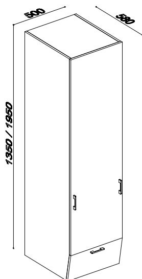
22092 LÉKÁRNA S VÝSUVNÝMI PLNÝMI DVÍŘKY 500 / 580 / 1350 MM
