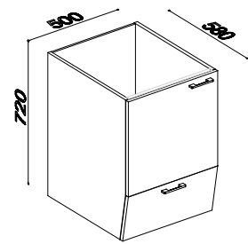
22011 SKŘÍŇKA SPODNÍ POD DŘEZ S DVÍŘKY
