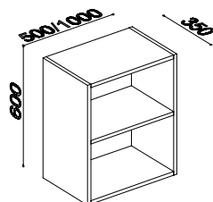
22026 SKŘÍŇKA HORNÍ POLICOVÁ 500 / 350 / 600 MM 22027 SKŘÍŇKA HORNÍ POLICOVÁ 1000 / 350 / 600 MM
