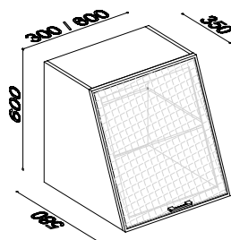
22075 NADSTAVEC NAD KARTOTÉKU A5 300 / 350-580 / 600 MM 22076 NADSTAVEC NAD KARTOTÉKU A5 600 / 350-580 / 600 MM
