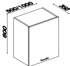
22028 SKŘÍŇKA HORNÍ S VÝKLOPNÝMI PLNÝMI DVÍŘKY 500 / 350 / 600 MM 22029 SKŘÍŇKA HORNÍ S VÝKLOPNÝMI PLNÝMI DVÍŘKY 1000 / 350 / 600 MM
