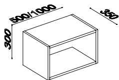
22020 SKŘÍŇKA HORNÍ POLICOVÁ 500 / 350 / 300 MM 22021 SKŘÍŇKA HORNÍ POLICOVÁ 1000 / 350 / 300 MM
