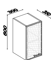
22036 SKŘÍŇKA HORNÍ SE SKLENĚNÝMI DVÍŘKY S AL. RÁMEČKEM
